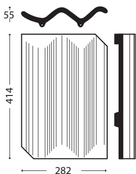
RT 804 Rød Højslev S-formet vingetegl
