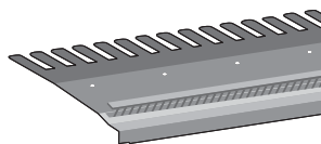
Højslev Tagfodselement Med fodblik, fuglegitter og ventilation: 200 cm 2 pr. lbm. mellem undertag og tagsten, 100 cm 2 pr. lbm. under undertag. Aluzink. Længde 100 cm. Dæklængde 98 cm. Aluzink. 100 cm lang.
