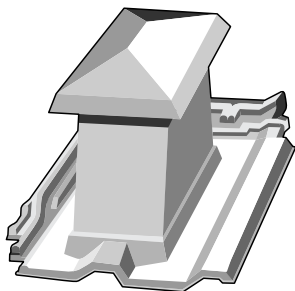
Udluftningshætte med isorør Tagvinkler Universal 20 - 45° Indvendig, ca. 150x150 mm Udluftning, ca. 225 cm 2
