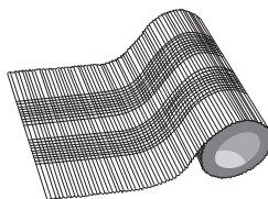
Gratbånd Alu med klæber og ventilation Farve Rød Bredde 320 mm Længde 500 cm Ventilationsareal 200 cm 2 pr. lb. m
