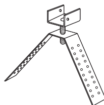
Toplægteholder Indstillelig, galvaniseret profil til montering af toplægte ved udluftning i tagrygning eller grat Antal i pakke ass.
