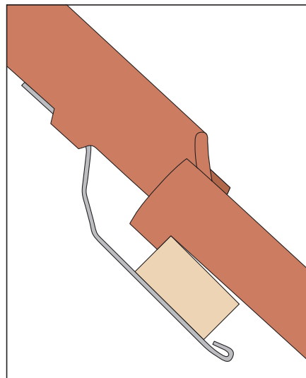
JP-takpannekrok
